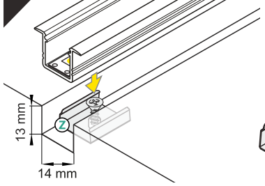
Z flexible mounting plate uchwyt Z sprężysty
